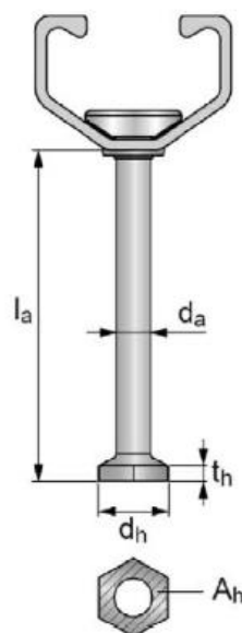
Приварний анкер
