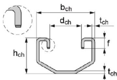
HAC-V-T 30
