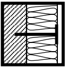
Кріплення утеплювача
