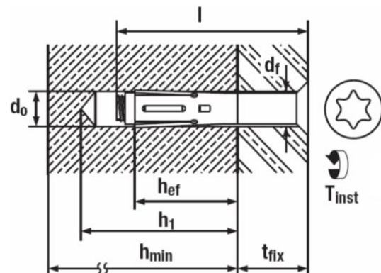
HLC-SK
