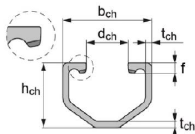
HAC-V-T 50, HAC-V-T 70
