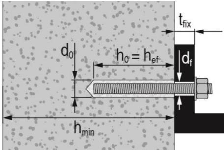
Повнотіла цегла з різьбовою шпилькою HIT-V або HAS-U або арматурою
