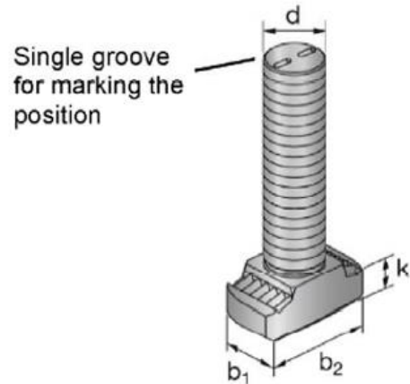
HBC-T
