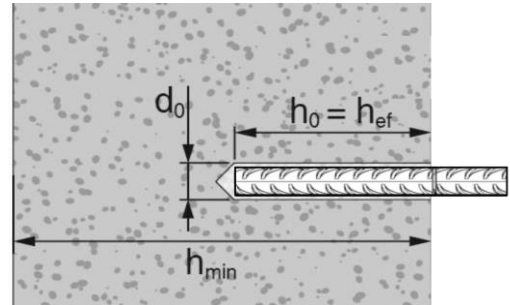
Повнотіла цегла з різьбовою шпилькою HIT-V або HAS-U або арматурою
