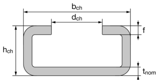
HAC-C 28/15, HAC-C 38/17
