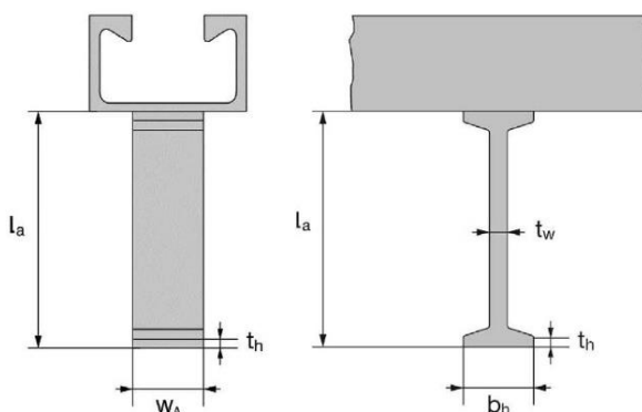
Варіант із привареним двотавровим анкером
