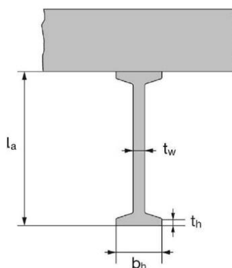
Варіант із привареним двотавровим анкером
