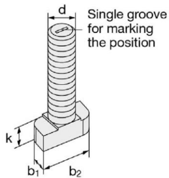
HBC-28/15, HBC-38/17
