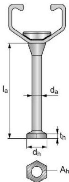
HAC-V з болтовим анкером
