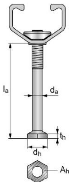
HAC з болтовим анкером
